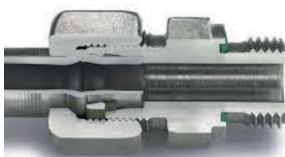
Parker E02 formmaskine Opfylder DIN EN ISO 8434-1 og er forhånds-godkendt af classeselskaber. Kan bruges til syrefast rør i størrelsen 12-38 mm S serie.
